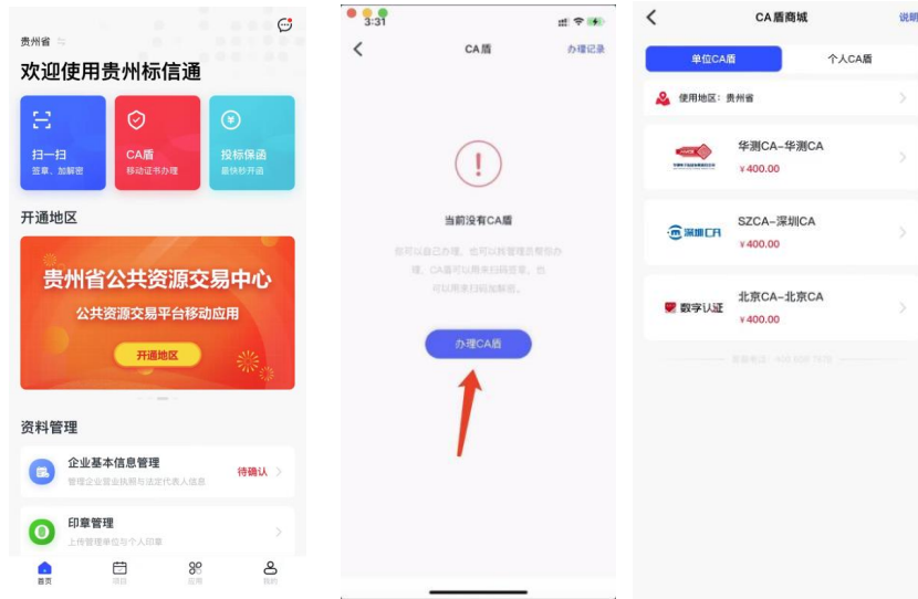
图 1.6.1 购买流程(1-3 步)
