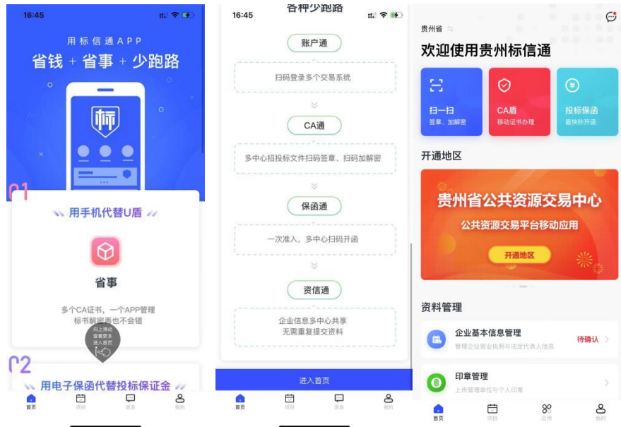
图 1.2.2 注册(6-7步)
